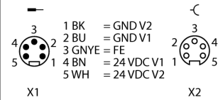
Napájecí konektor 7/8"
