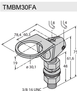
Montážní úchytka, nerez, pro 30mm závit
