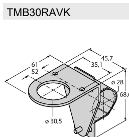
Montážní úhelník, nerez, pro senzory v závitových pouzdrech M30, pro montáž na kruhové tyče o průměru 28 mm
