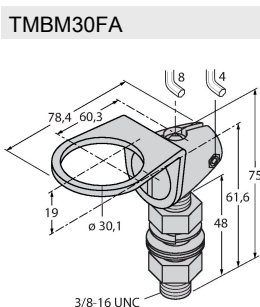
TMBM30FA 7700398 Uchwyt montażowy, stal nierdzewna, dla gwintu 30 mm
