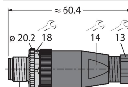
M12 x 1
