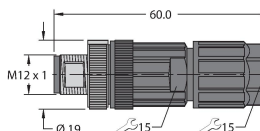
M12 x 1
